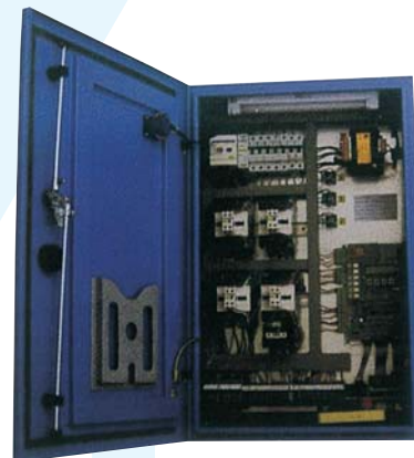
Çift hızlı ve VVVF Asansörler için kumanda panoları
